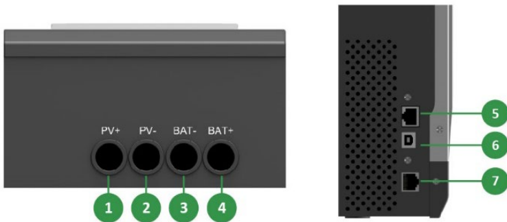
Esquema de conexión
