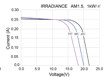
Curvas I-V del módulo PV ESF-5PA a varias temperaturas de célula I-V Curves of PV module ESF-5PA at various cell temperatures
