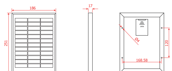
Dimensiones - Dimensions ESF-5PA
