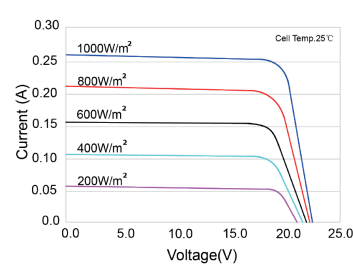
Curvas I-V del módulo PV ESF-5PA I-V Curves of PV module ESF-5PA
